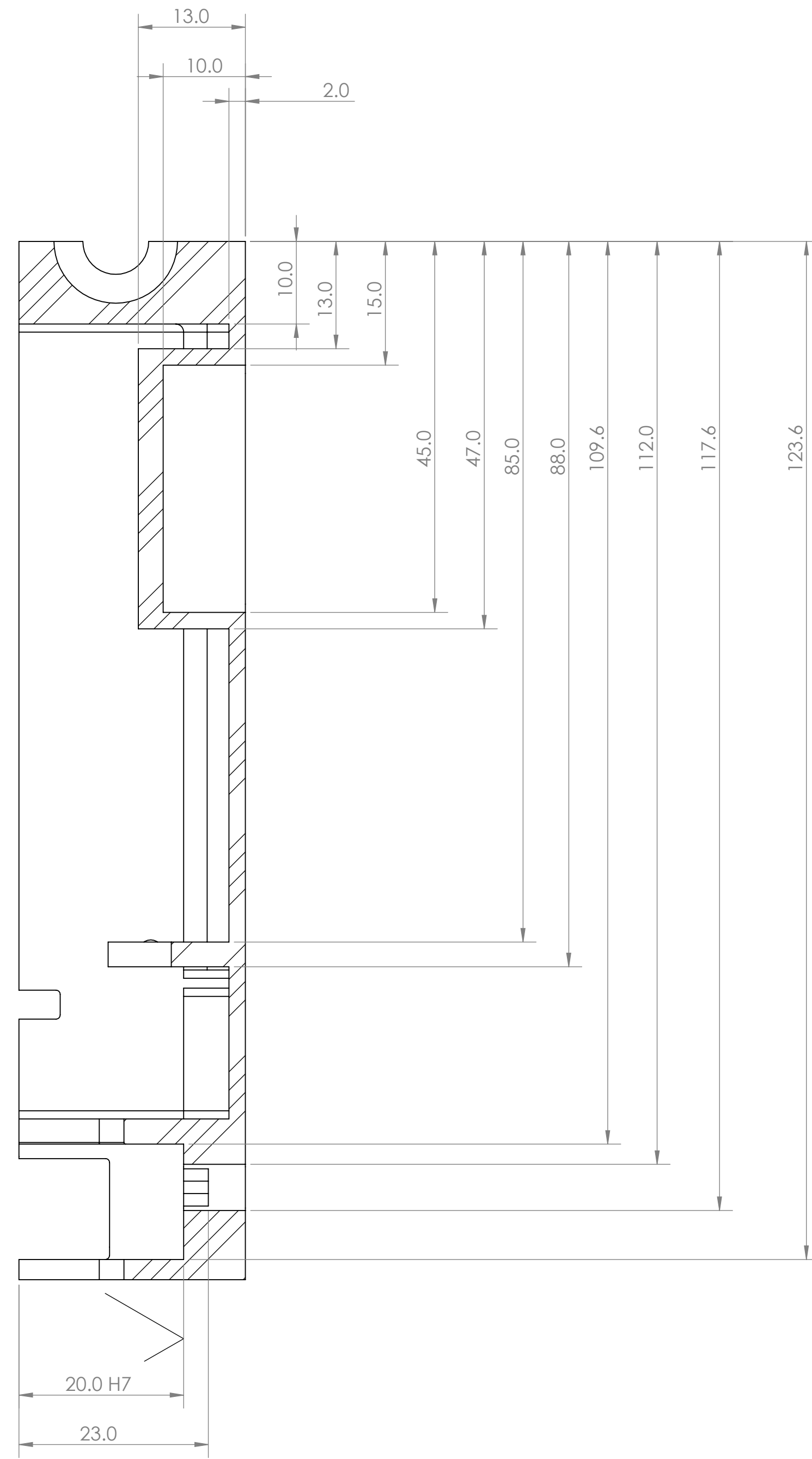
SECTION A-A
